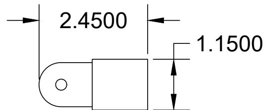
Rod End
